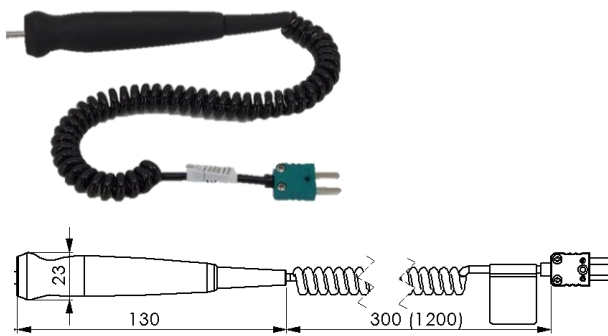
volitelně spirálový kabel CC12
